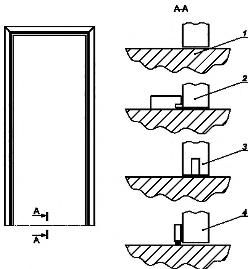
1 — без порога; 2 — с приставным порогом; 3 — с выдвижным порогом встраиваемого типа; 4 — с выдвижным порогом накладного типа
