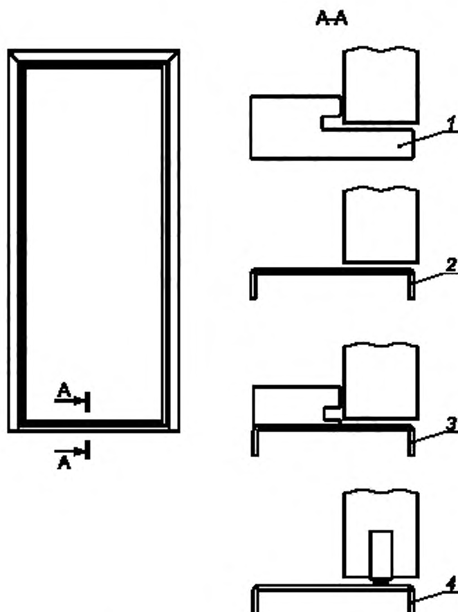
Рисунок А.4 — Примеры конструктивного исполнения дверей с замкнутой коробкой
